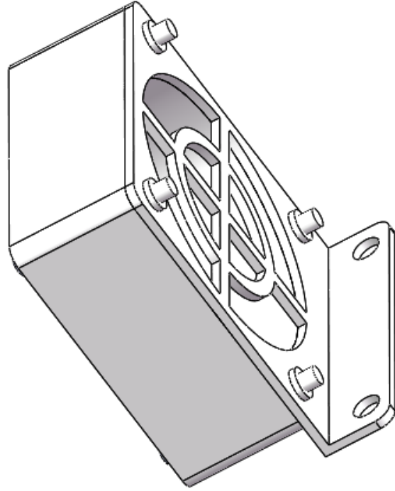
20.205.0099 主板散热风扇组件 Motherboard Cooling Fan Assembly
